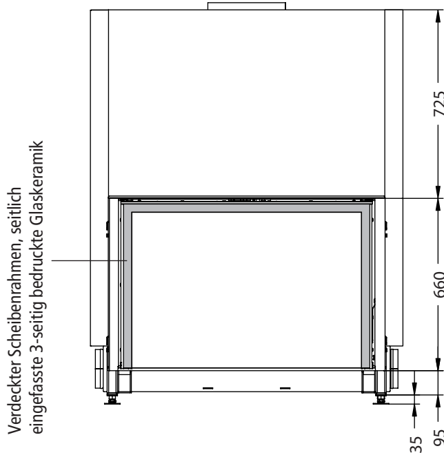
Vorderansicht M~1:20
